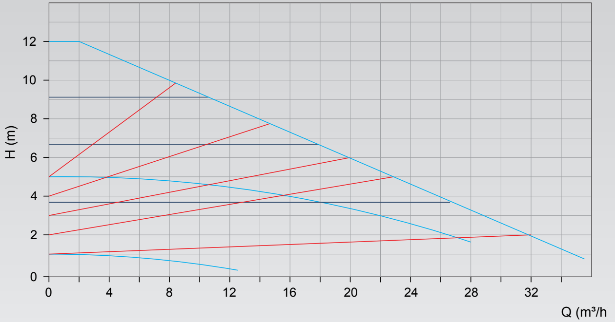
ECP50-180F
