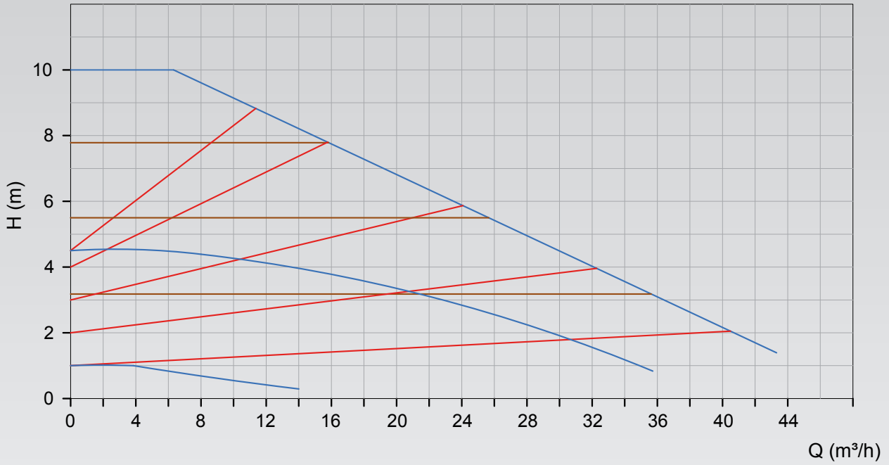
ECP65-100F
