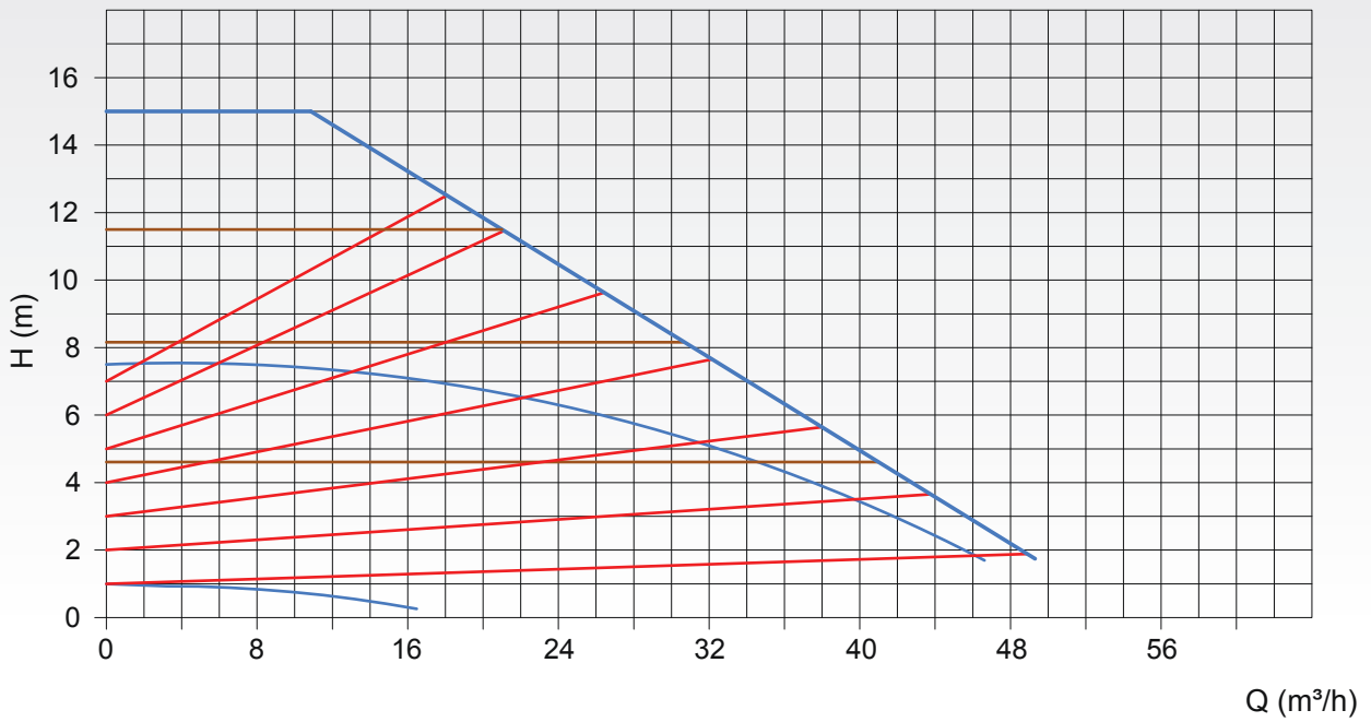
ECP65-150F
