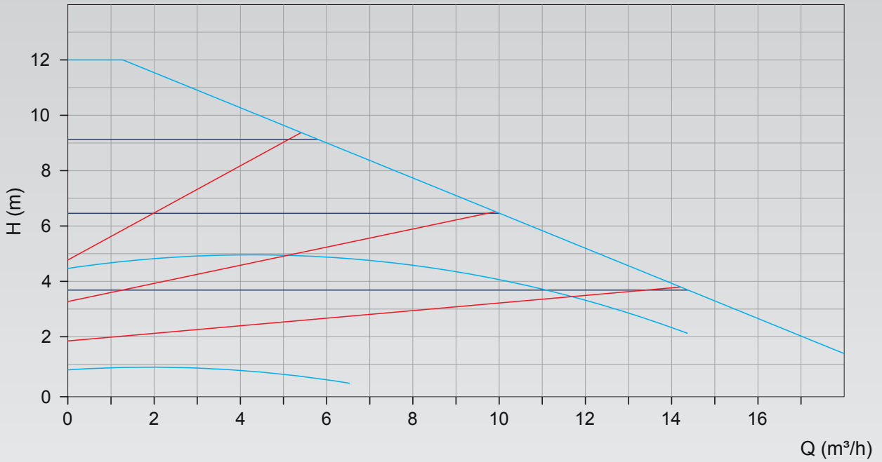
ECP32-120F
