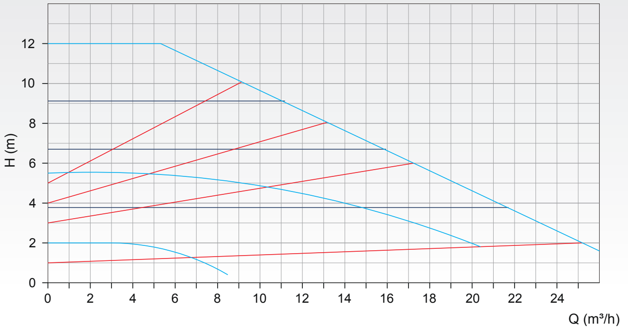
ECP40-120F
