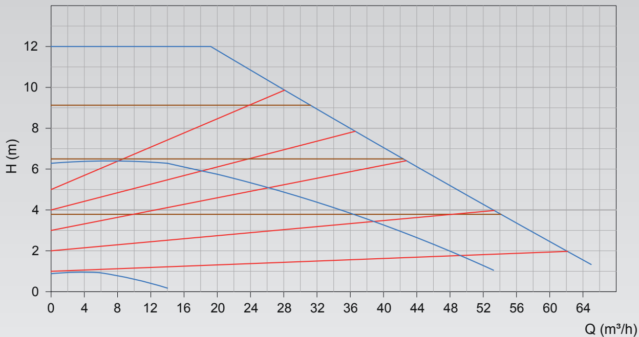
ECP80-120F
